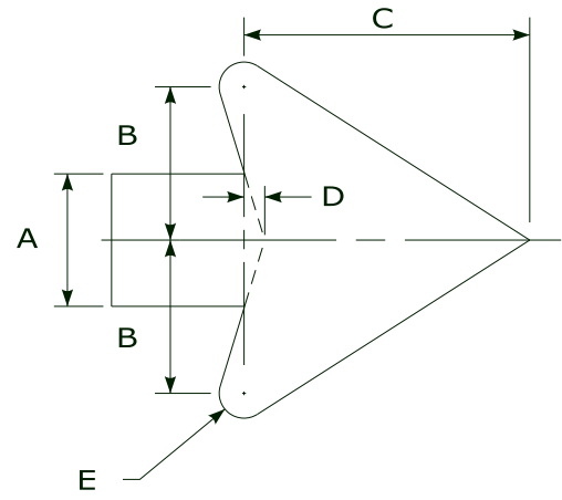
ARROWHEAD D15 DETAIL N.T.S.
