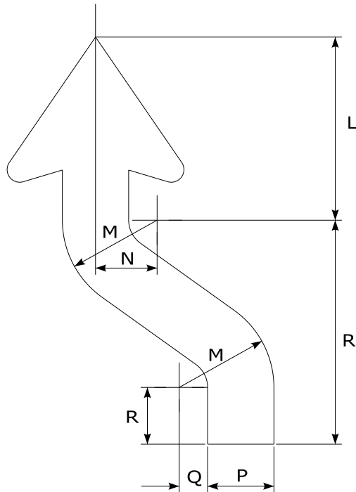
ARROW DETAIL N.T.S.
