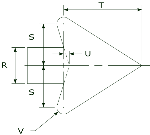
ARROWHEAD DETAIL N.T.S.
