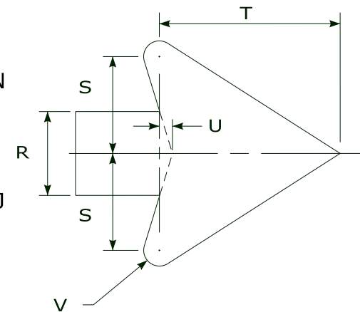
ARROWHEAD DETAIL N.T.S.
