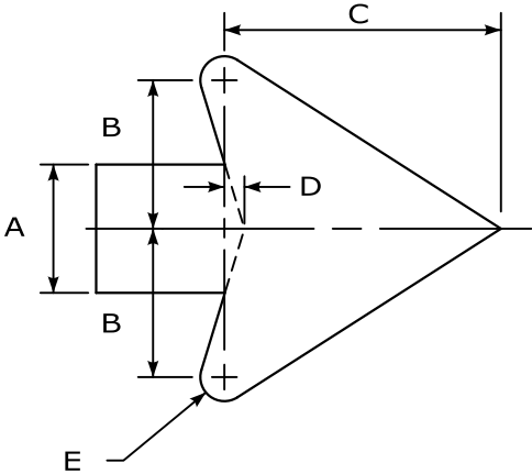
ARROWHEAD D-6 DETAIL N.T.S.
