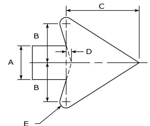
ARROWHEAD D-6 DETAIL N.T.S.
