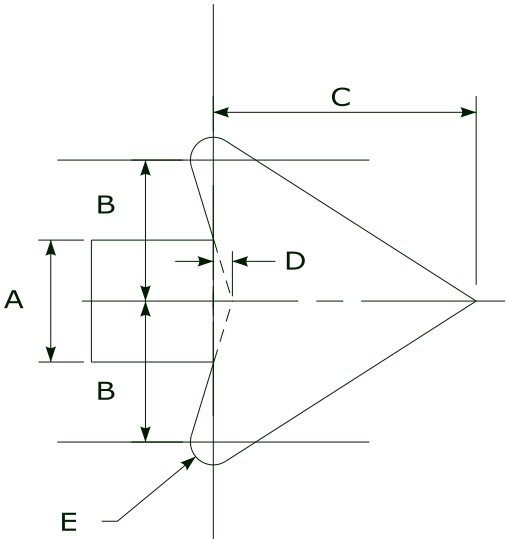
ARROWHEAD D-6 DETAIL N.T.S.
