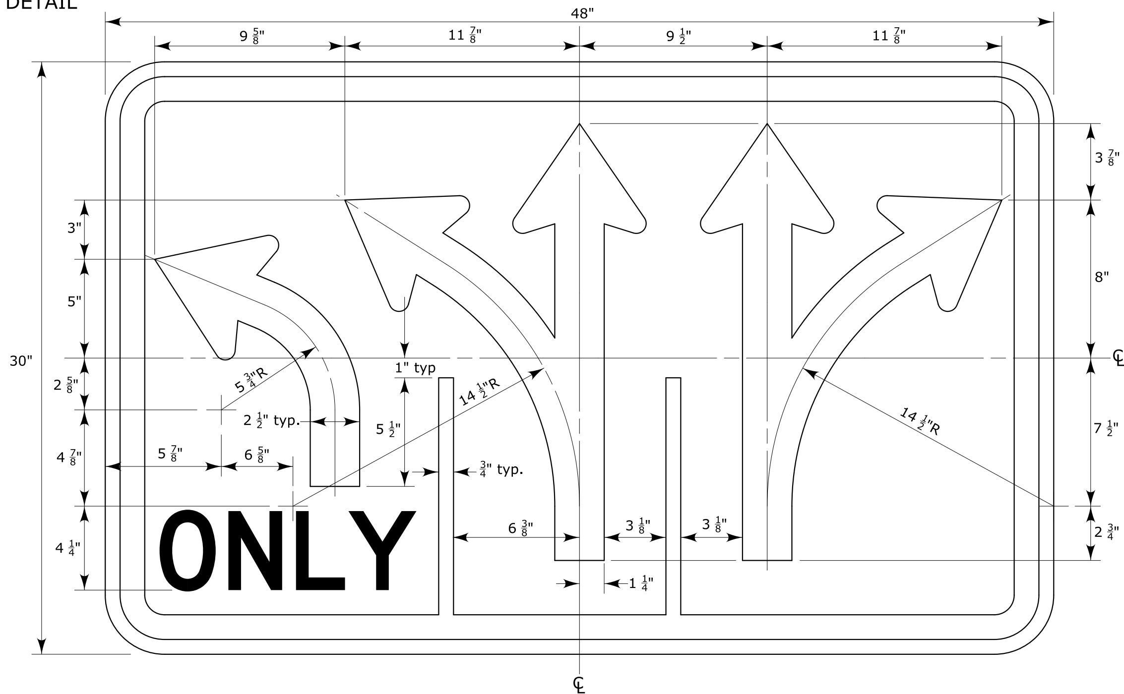
ARROWHEAD D-6 DETAIL N.T.S.
