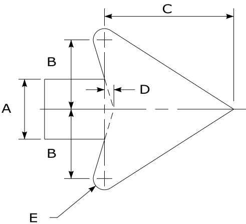
ARROWHEAD D-6 DETAIL N.T.S.
