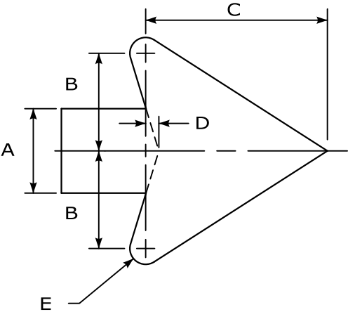
ARROWHEAD D-6 DETAIL N.T.S.
