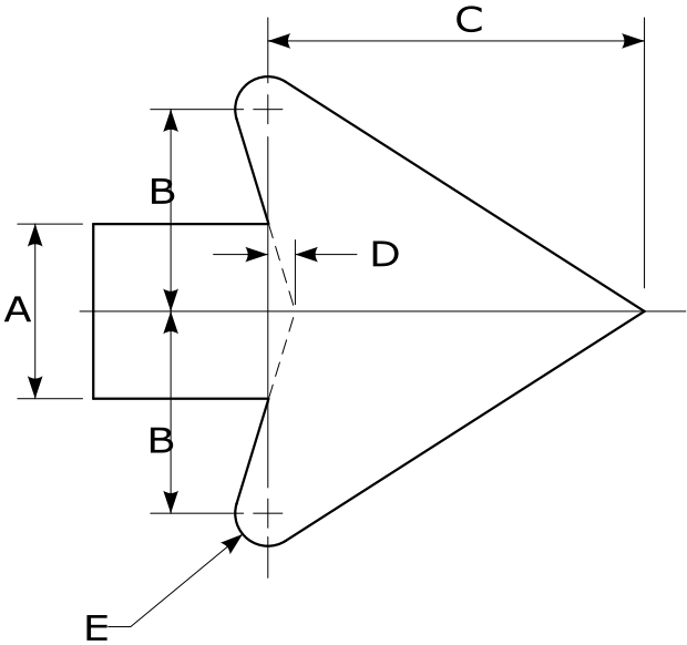
ARROWHEAD DETAIL N.T.S.
