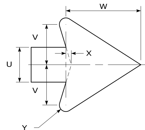
ARROWHEAD DETAIL N.T.S.
