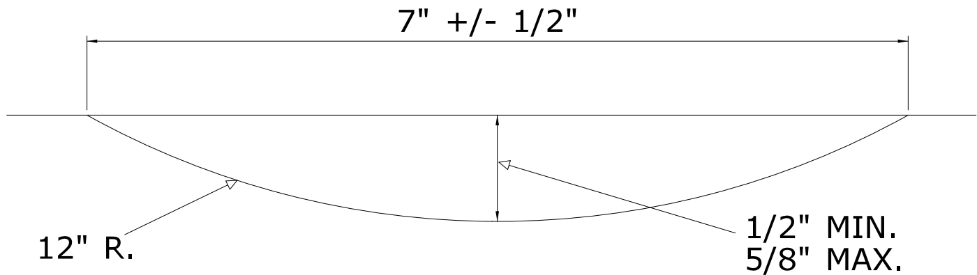
SECTION A-A
